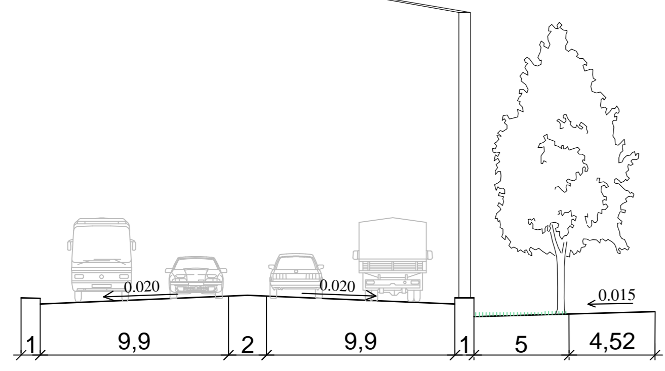
Розріз 1-1 М1:100
