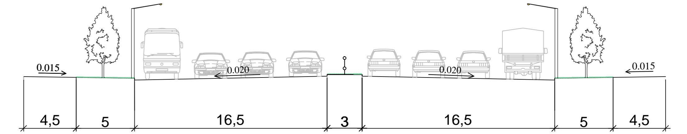
Поперечний профіль вул. Академіка Заболотного М1:100
