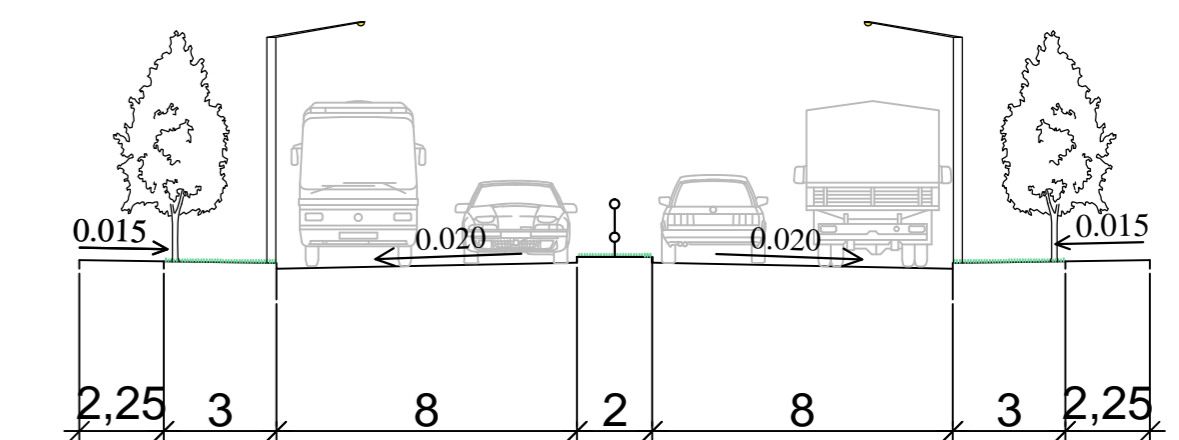
Поперечний профіль вул. Івана Сірка М1:100
