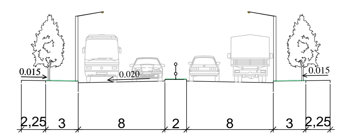
Поперечний профіль вул. Івана Сірка М1:100
