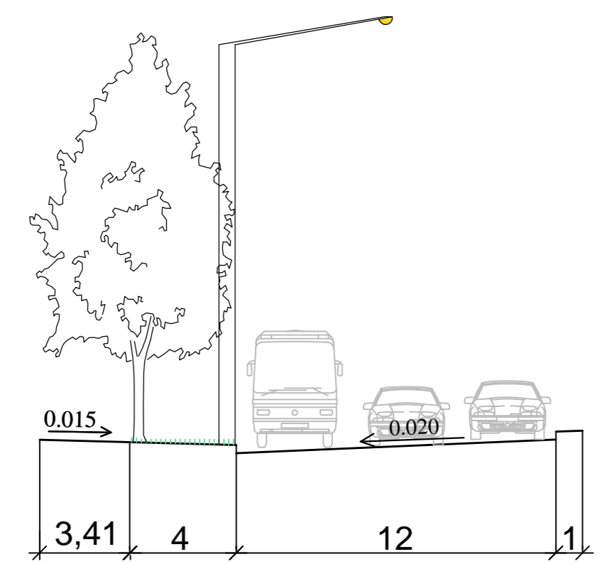
Розріз 3-3 М1:100 вул. Івана Сірка
