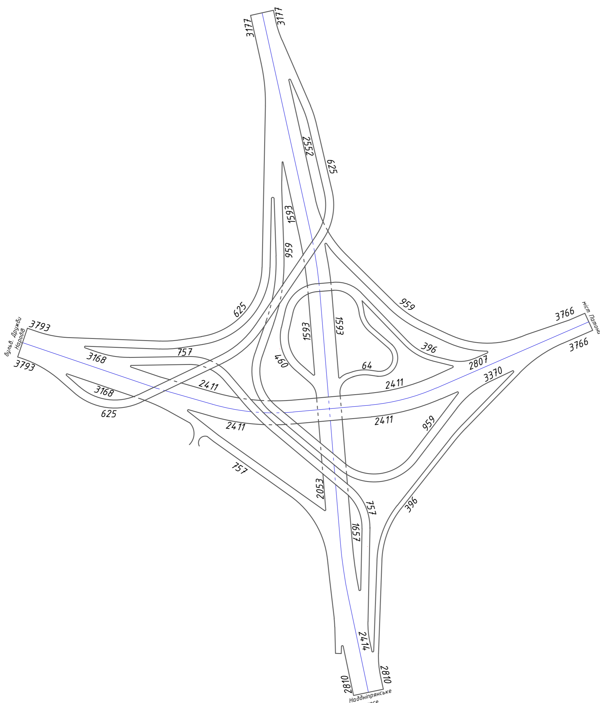
Інтенсивності руху на окремих ділянках вузла
