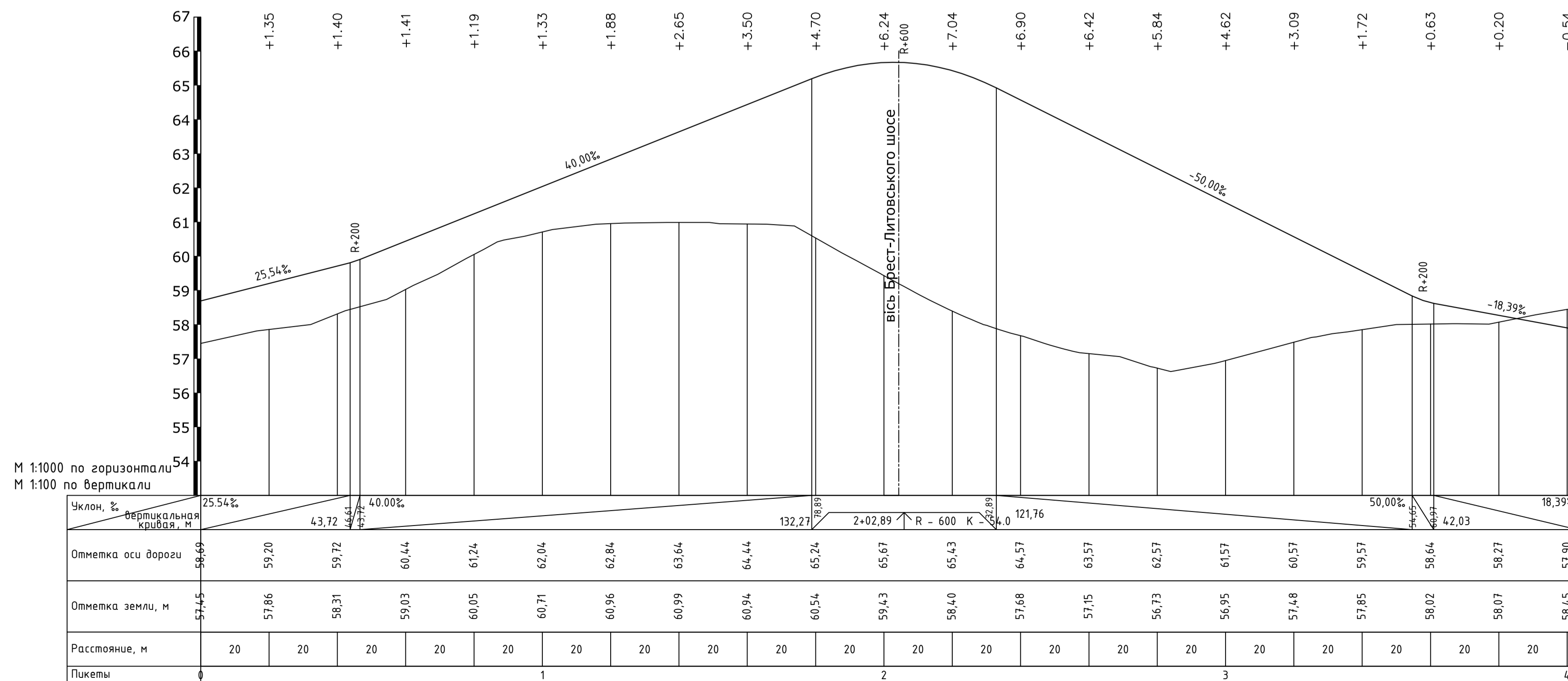
Лівоповоротний з'їзд 4-2
